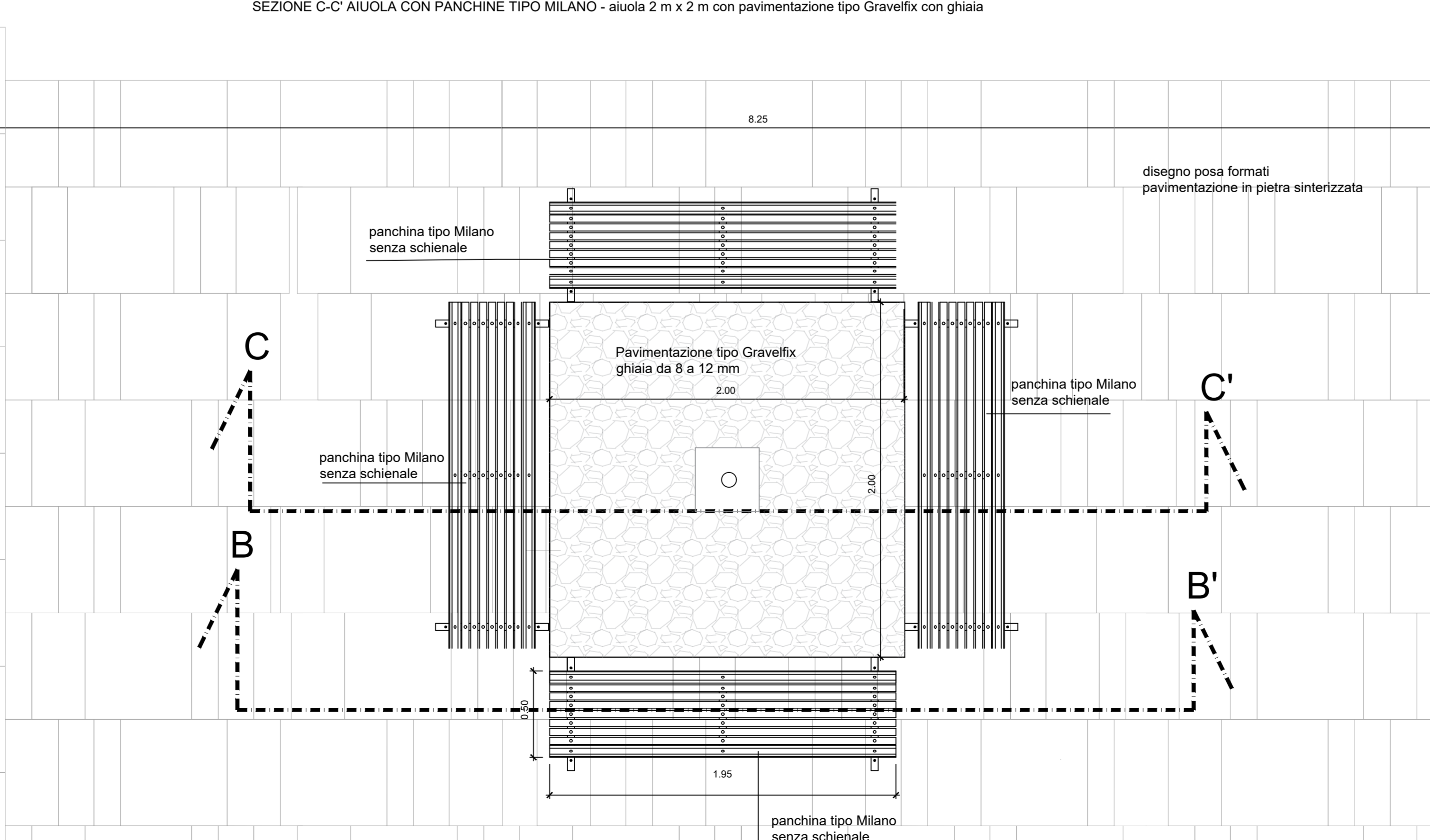
DETTAGLI POSA PANCHINE-TAVOLI TIPO MILANO - SDP_NUOVA PIAZZA PAPA GIOVANNI XXIII (1:20)
