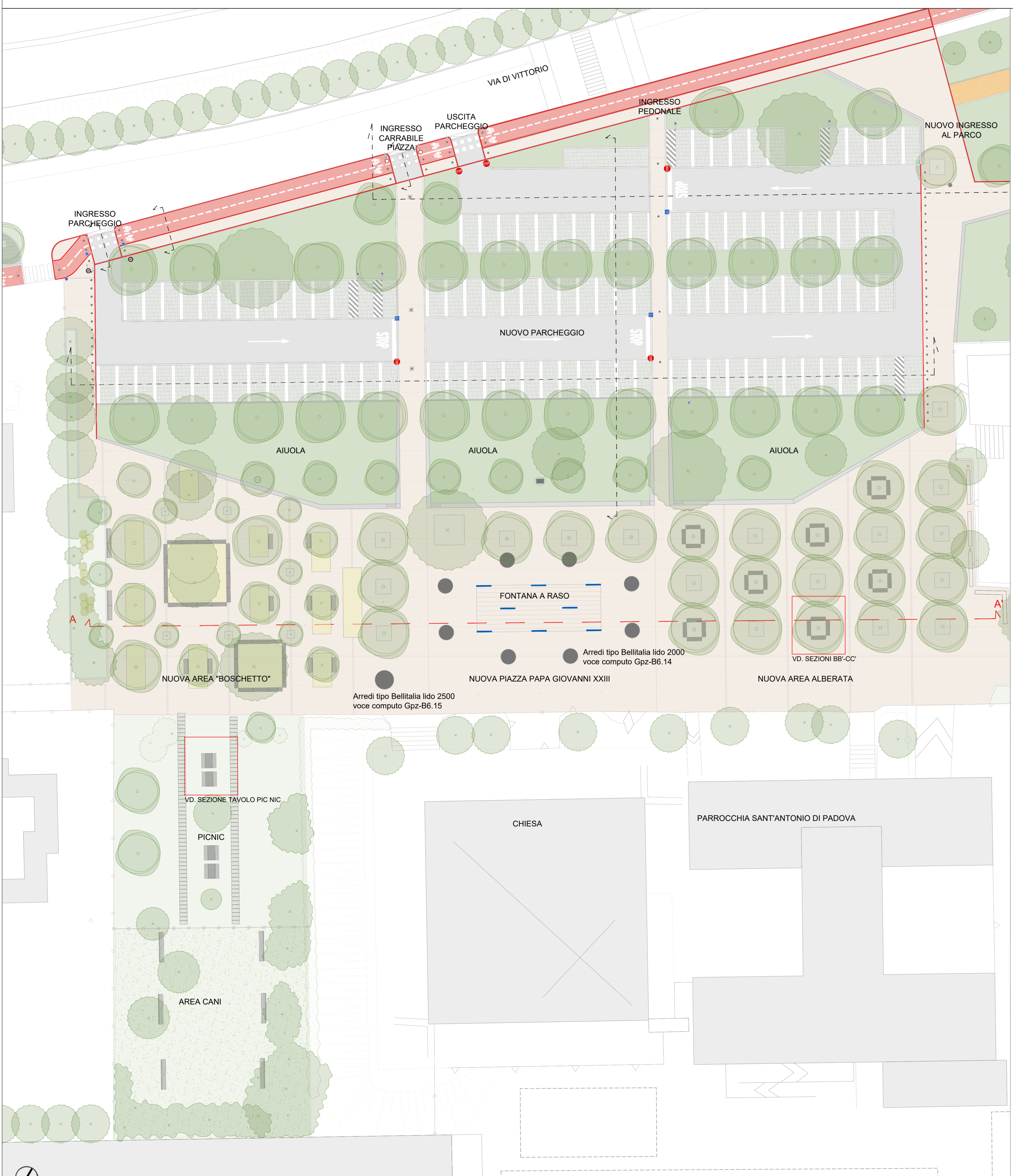
PLANIMETRIA GENERALE - SDP_NUOVA PIAZZA PAPA GIOVANNI XXIII E PARCHEGGIO (1:250)
