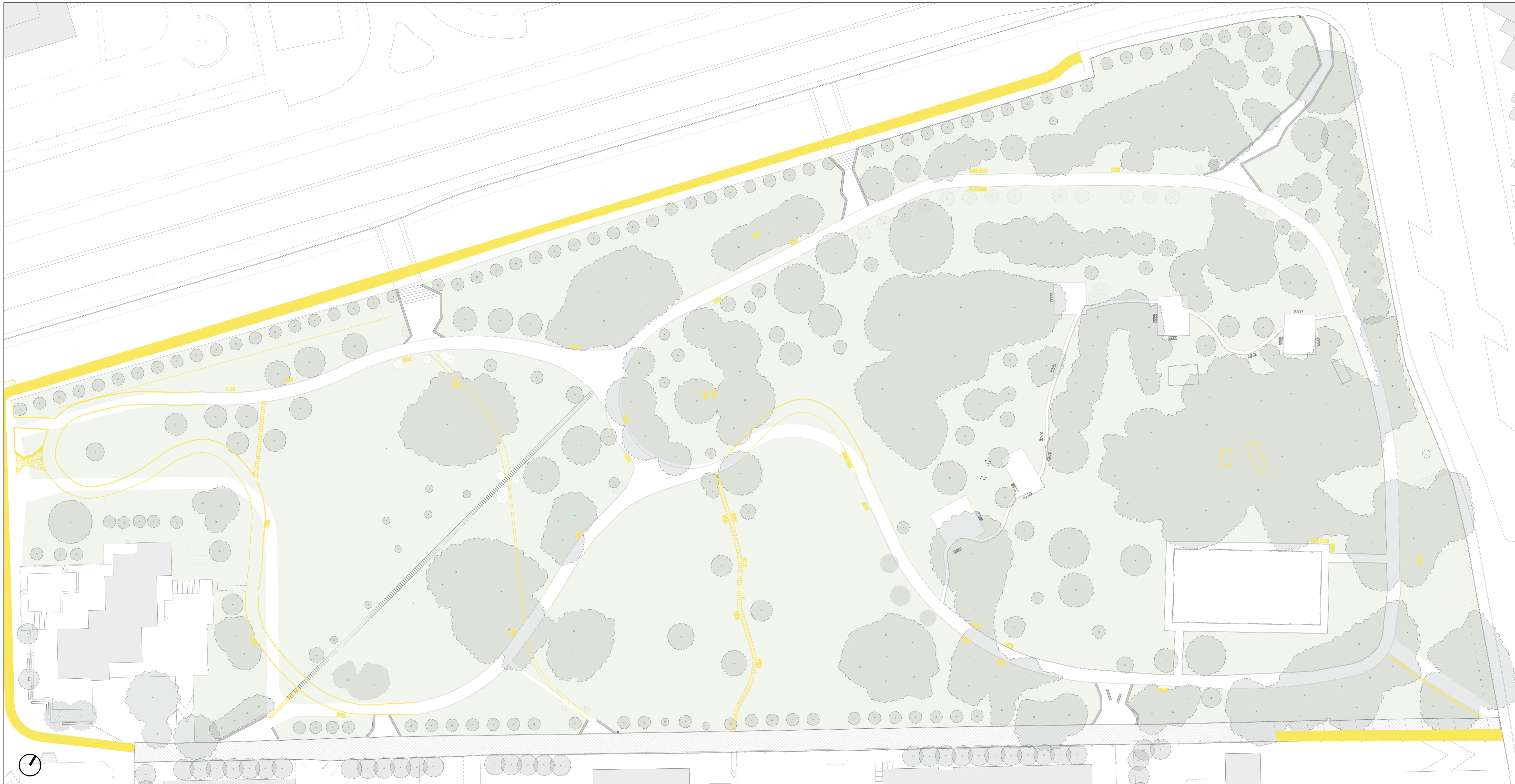
PLANIMETRIA GENERALE - STATO DI CONFRONTO GIALLI DEMOLIZIONI PARCO GIORGELLA - SCALA 1:450
