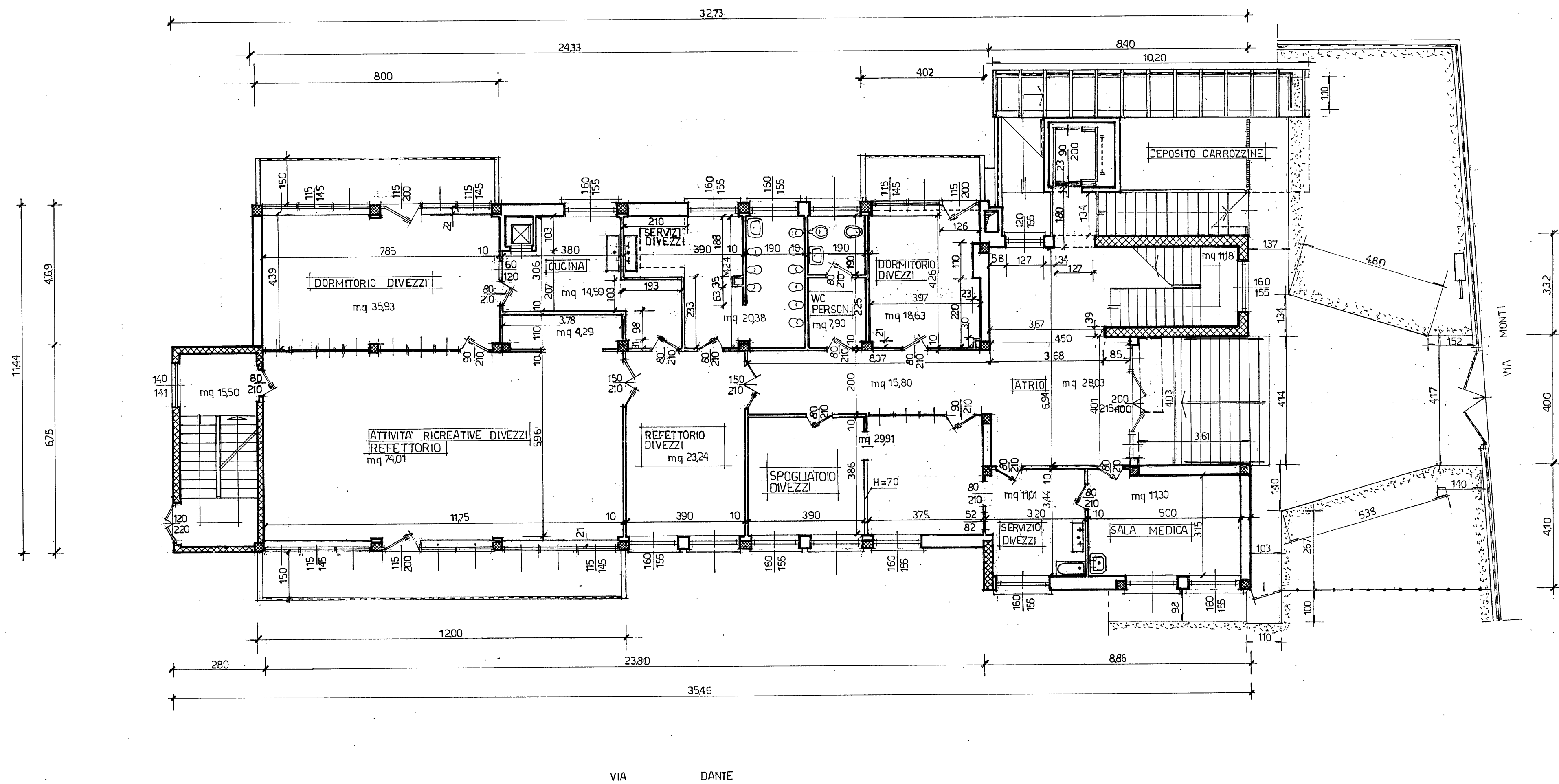
PIANTA PIANO RIALZATO SCALA 1/100
